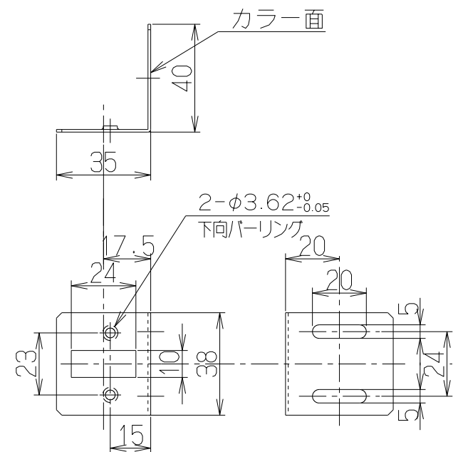
取付ベース
