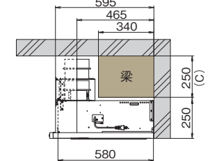
背梁の場合
