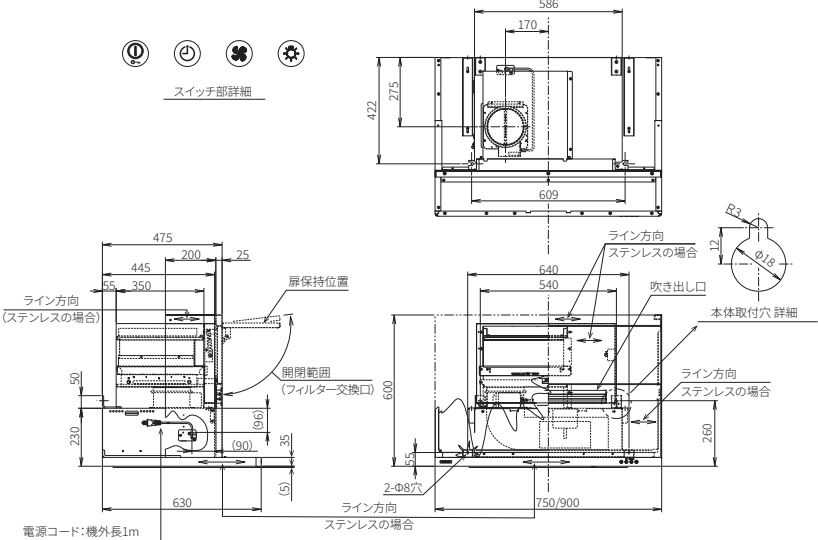
【製品寸法図】
