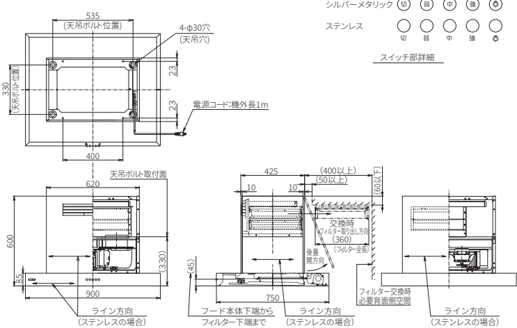
【製品寸法図】
