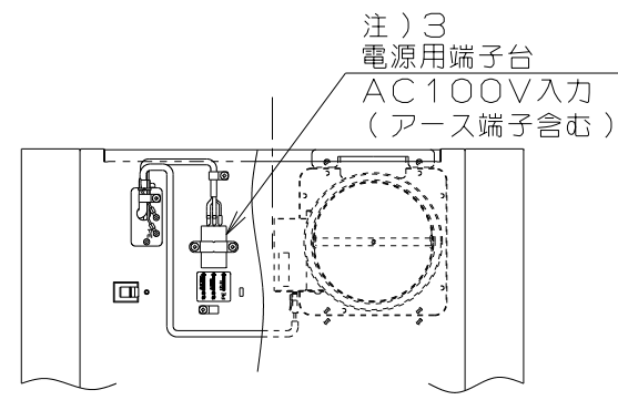
×矢視図
