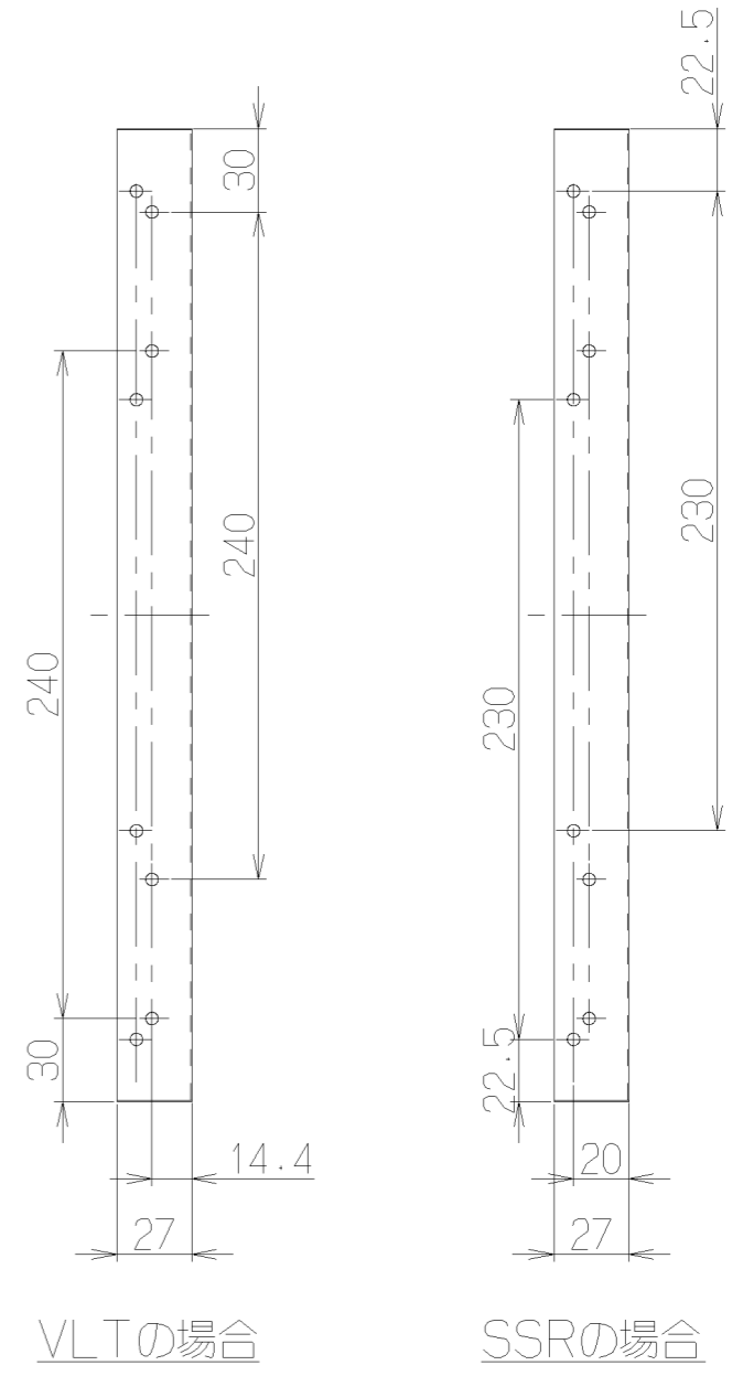
使用取り付け穴詳細
