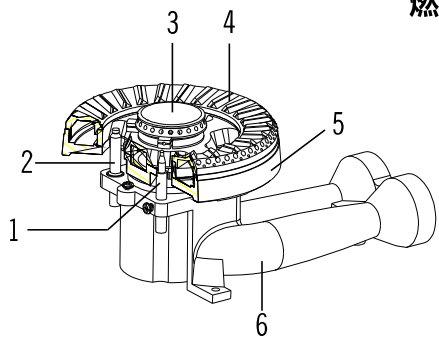
主燃烧器
