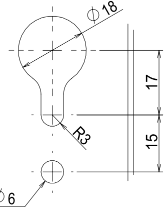
Detail:Installation hole
