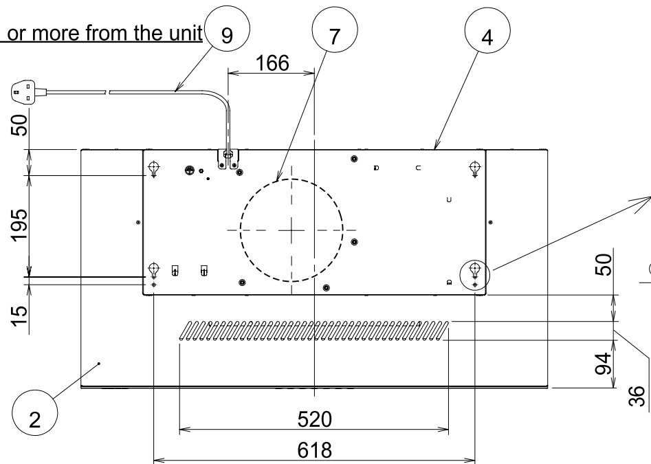
Detail:Installation hole
