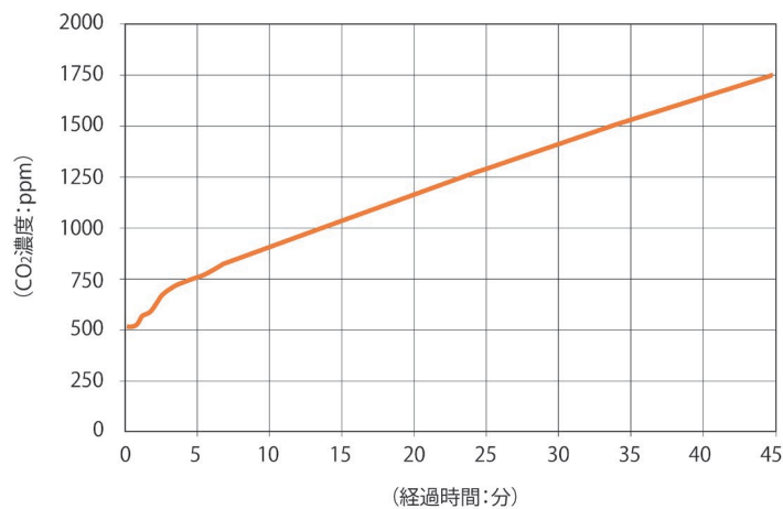
石油ファンヒーター稼働中の部屋の CO 2 濃度の推移
