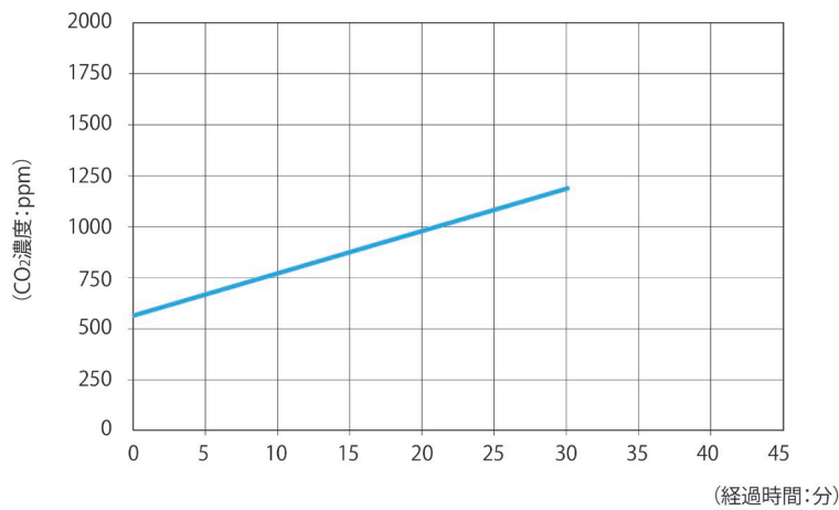
成人男性 4 人相当、16 畳の部屋中央で着座事務作業をした際の CO 2 濃度の推移
